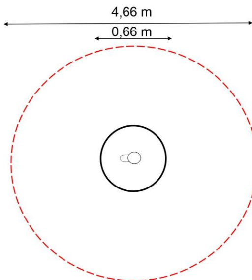
KARUZELA KTR-08 | STREFA BEZPIECZEŃSTWA
