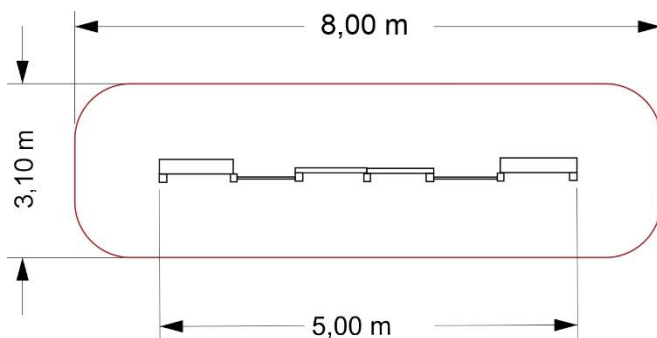
STREFA BEZPIECZEŃSTWA | ZU2
