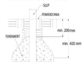
SYSTEM MONTAŻU SŁUPA METALOWEGO W BETONIE
